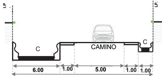
SECCION EXISTENTE SECCION D-D
