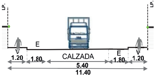
SECCION PROPUESTA SECCION B-B
