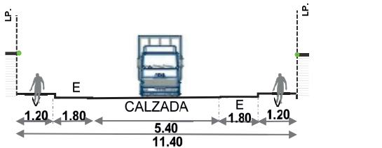
SECCION PROPUESTA SECCION C-C y D-D
