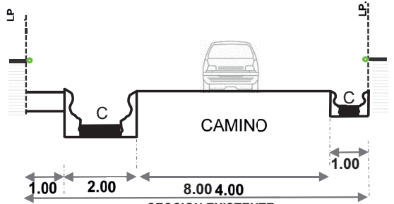
SECCION EXISTENTE SECCION C-C
