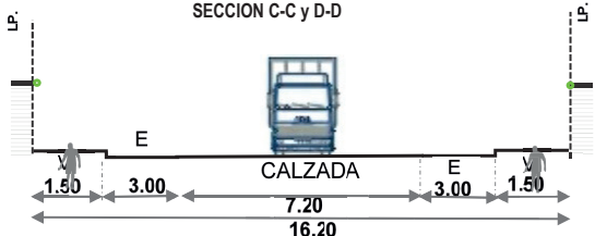
ANTIGUA PANAMERICANA SUR SECCION A-A
