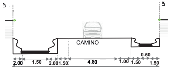
SECCION EXISTENTE SECCION B-B
